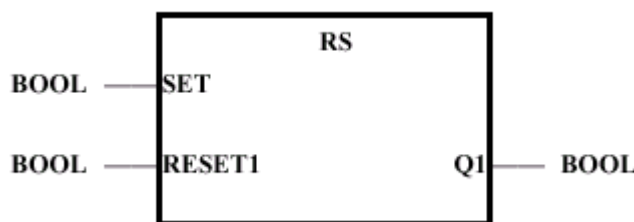
6. ábra RS-tároló
