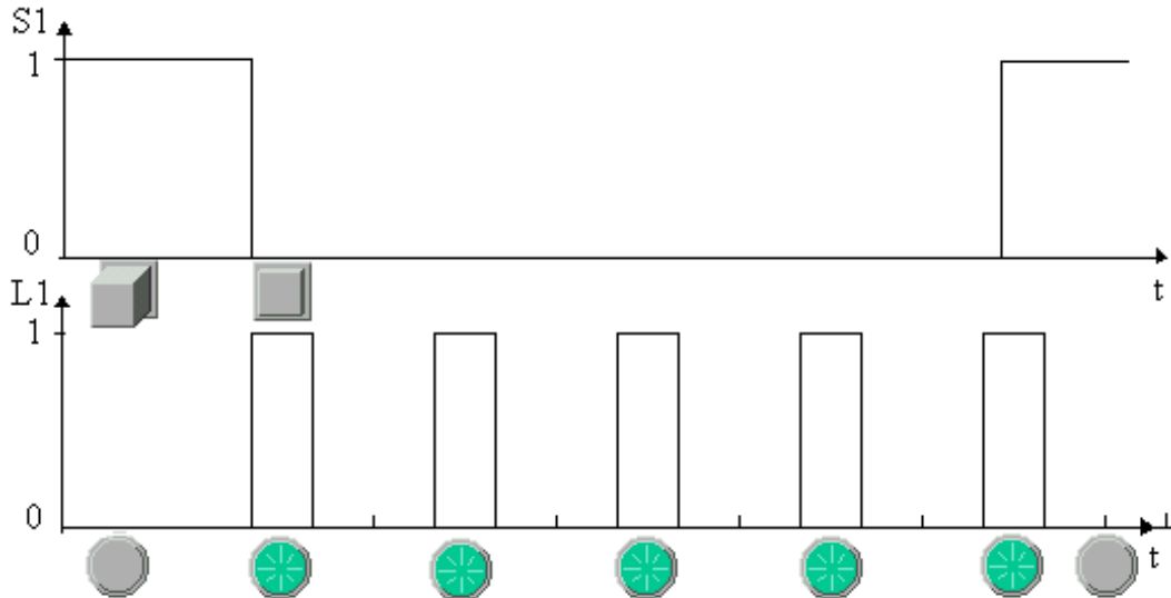
29. ábra Idődiagram
